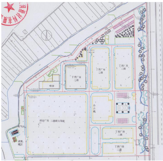
图 3.4 平面布局图
